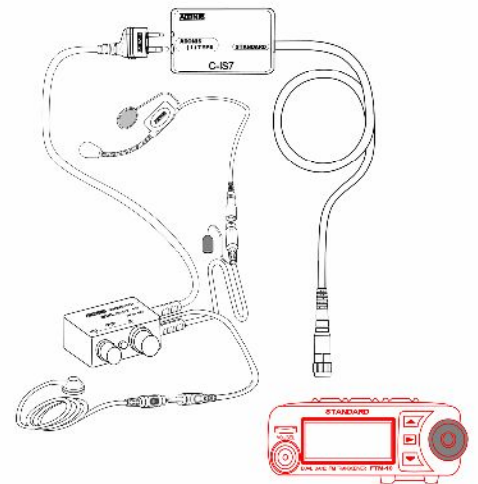
C - I S 7 配線例 ( 2 図 )
